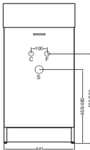
VISTA FRONTALE
