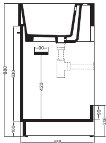
SEZIONE B-B
