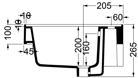
SEZIONE A-A'
