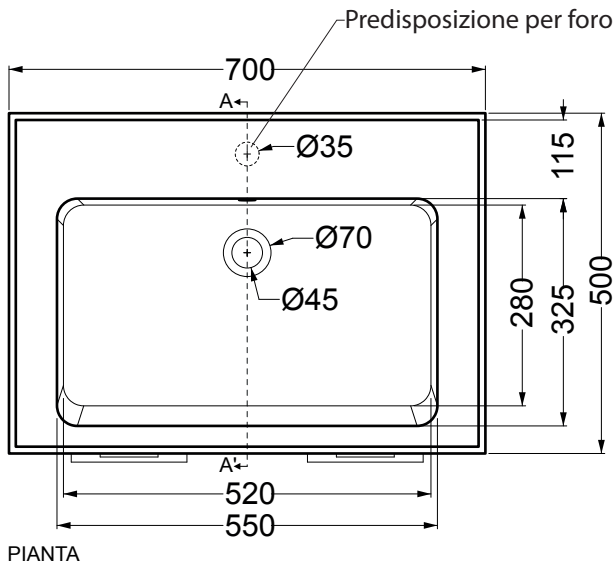
PIANTA
