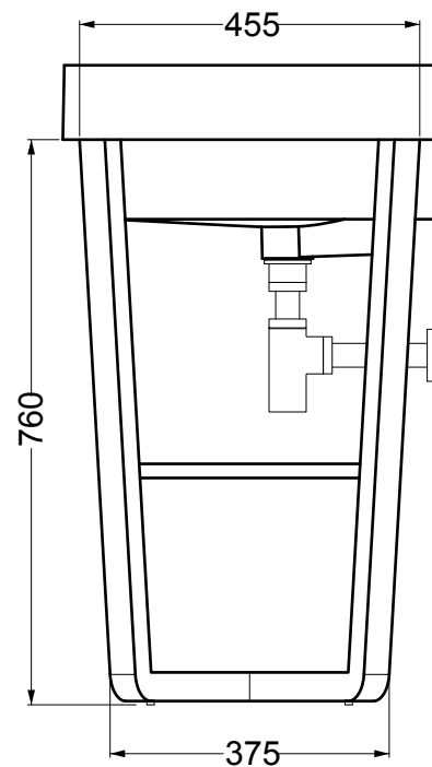
VISTA LATERALE
