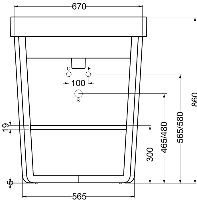
VISTA FRONTALE
