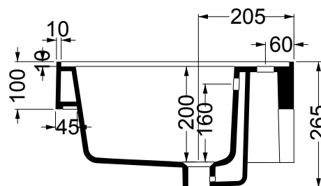
SEZIONE A-A'
